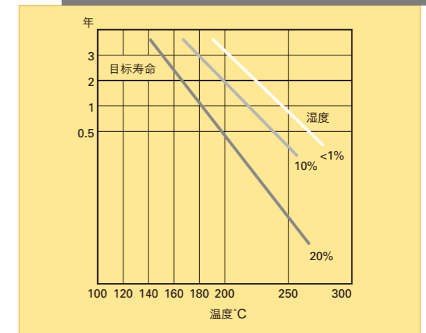
图10：水份及温度对杜邦™ Nomex® 纤维滤袋的影响
