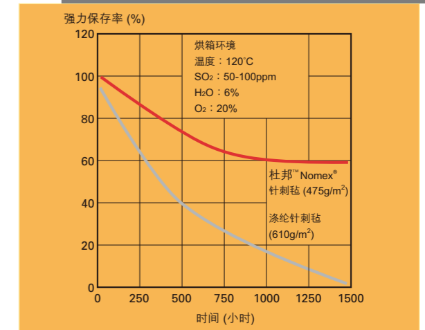
图9：杜邦™ Nomex® 布及涤纶布在 120°C 下其强度的比较
