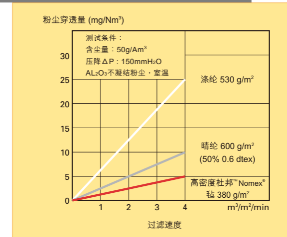
图8：杜邦™ Nomex® 无纺布的除尘效率
