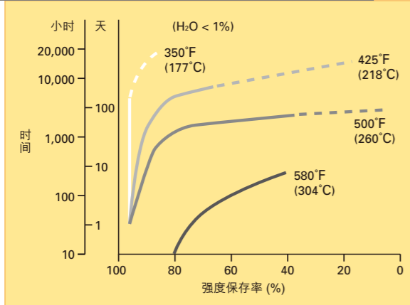
图5：杜邦™ Nomex® 纤维在热空气中的强度保存率
