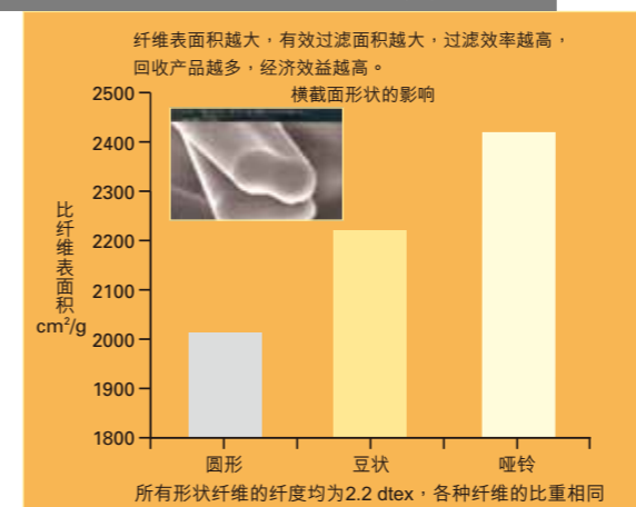
图4：杜邦™ Nomex® 针刺毡的过滤效率(续)
