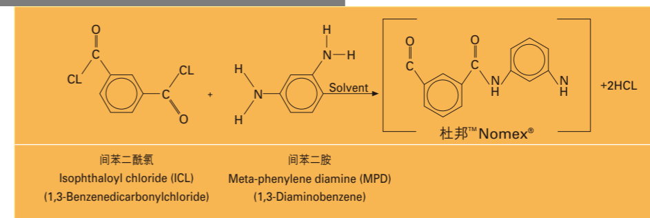
图3：杜邦™ Nomex® 纤维的合成反应
